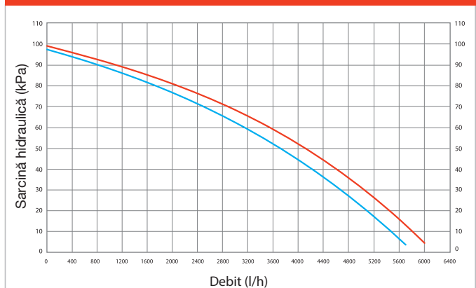
Grafic debit / sarcină hidraulică VICTRIX PRO 120
