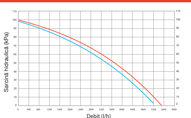
Grafic debit / sarcină hidraulică VICTRIX PRO 100
