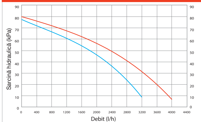
Grafic debit / sarcină hidraulică VICTRIX PRO 80
