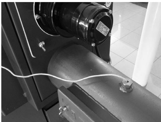
Fig. 14 – imaginea senzorului de gaze de ardere TS în recipientul canalului de fîp
