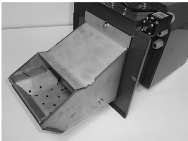
Fig. 1 – duza de ardere a arzătorului
