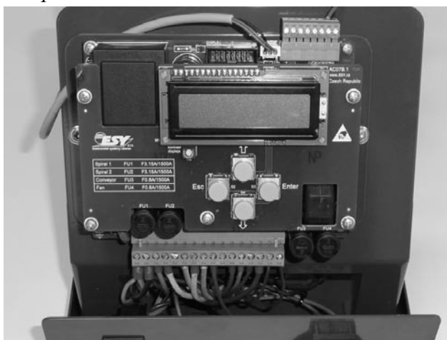
Fig. 5 – unitate electronică de comandă cu butoane, cutia de borne inferioară (1-18), cutia de borne superioară pentru conectarea senzorilor TS (poziția 3 și 4) și TV (poziția 6 și 7)
